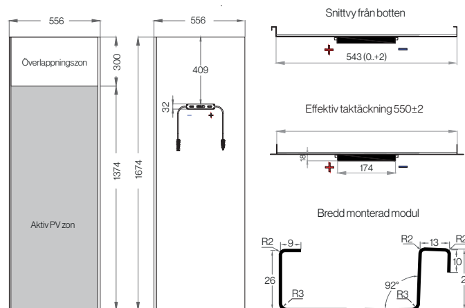
Konstruktionsritningar (mm)
