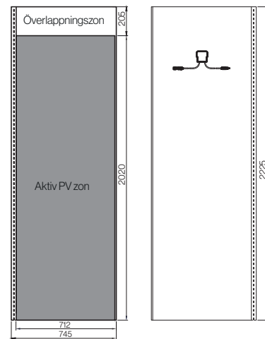
Konstruktionsritningar (mm)
