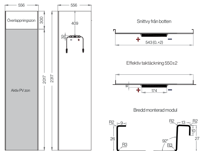
Konstruktionsritningar (mm)
