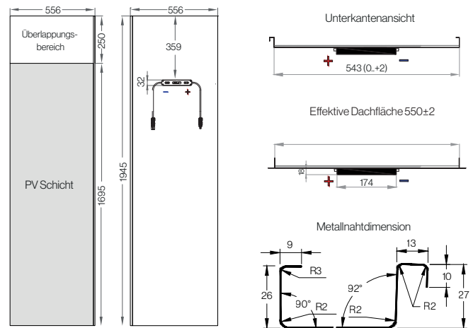
Konstruktionszeichnungen (mm)
